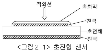
<그림 2-1> 초전형 센서
